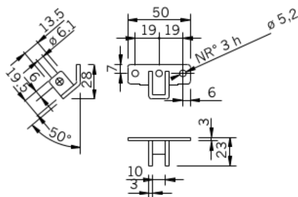
CD97004400 Kabelová příponka
