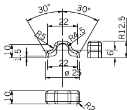
CD97004400 Kabelová příponka
